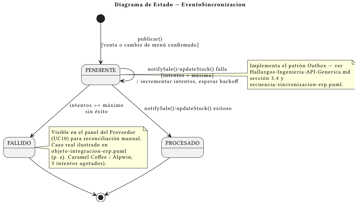
Figura 13: Estado: EventoSincronizacion
